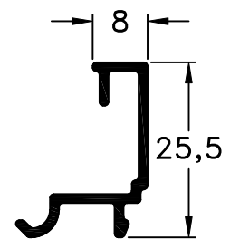
879 - Contravidrio peso: 0,21 Kg/m
