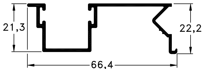
722 - Guía de Cortina Común Largo Std.: 6150 mm Peso: 0,49 Kg/m
