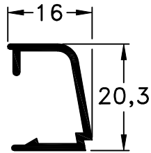
523 - Contravidrio peso: 0,17 Kg/m
