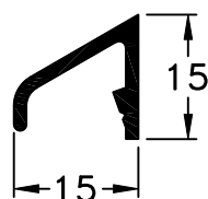
200 - Bota-Agua peso: 0,15 Kg/m
