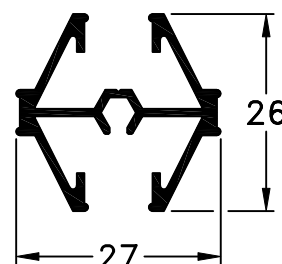
471 - Travesaño peso: 0,36 Kg/m
