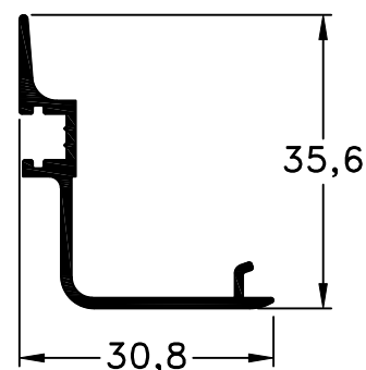
26 - Encuentro Hoja peso: 0,27 Kg/m
