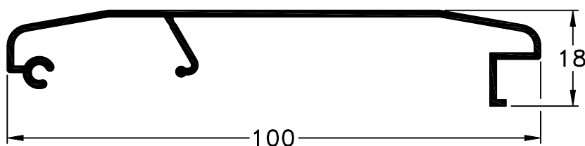
716 - Tapacinta Largo Std.: 6150 mm peso: 0,52 Kg/m
