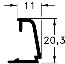
705 - Contravidrio peso: 0,16 Kg/m
