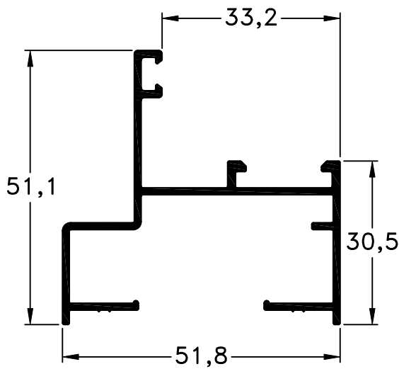
75 - Marco Paño Fijos y Ventana Doble Contacto Largo Std.: 6150 mm peso: 0,64 Kg/m
