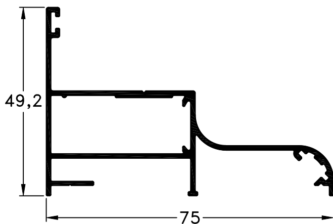
485 - Marco peso: 0,77 Kg/m
