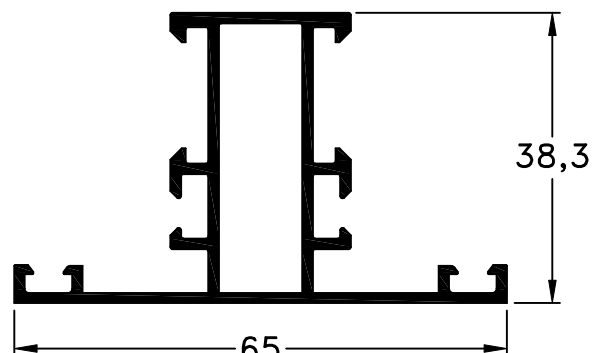
733 - Travesaño peso: 0,81 Kg/m
