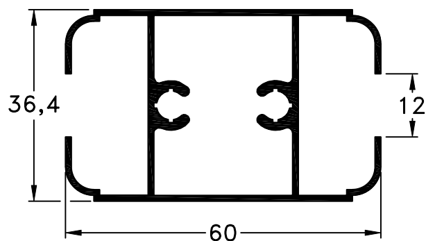
552 - Travesaño peso: 0,86 Kg/m
