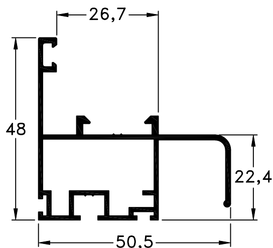
506 - Zócalo/Cabezal peso: 0,69 Kg/m
