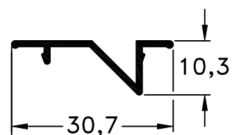
509 - Tapa peso: 0,14 Kg/m
