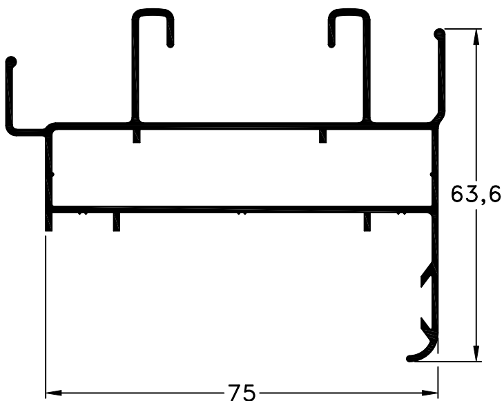
489 - Marco con Contramarco Largo Std.: 6300 mm peso: 1,06 Kg/m
