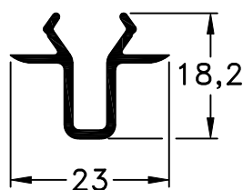
27 - Encuentro 4 Hojas para Perfil 481 y 482 peso: 0,18 Kg/m
