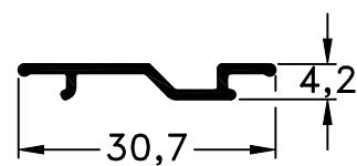
129 - Tapa Doble Compensador peso: 0,12 Kg/m
