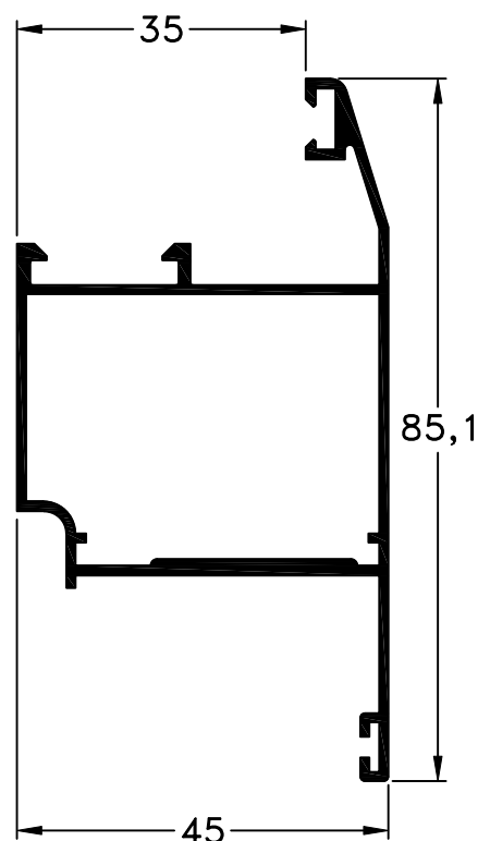
737 - Hoja peso: 0,83 Kg/m
