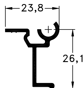
750 - Soporte Tapacinta Largo Std.: 6150 mm peso: 0,28 Kg/m
