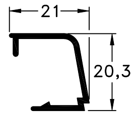
706 - Contravidrio peso: 0,20 Kg/m
