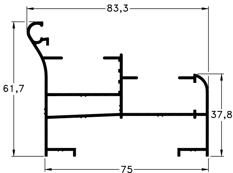
505 - Marco Ventana Guillotina peso: 0,97 Kg/m
