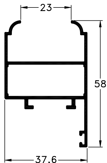
21 - Hoja peso: 0,65 Kg/m
