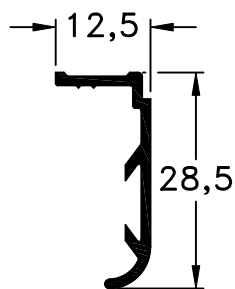
487 - Contramarco Largo Std.: 6150 mm peso: 0,17 Kg/m
