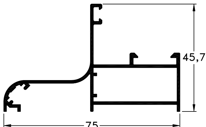
516 - Marco Largo Std.: 6150 mm peso: 0,76 Kg/m
