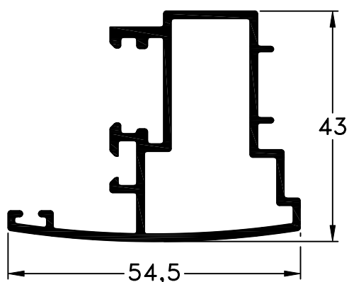
702 - Inversor Hoja peso: 0,81 Kg/m
