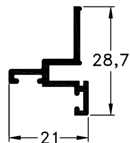
725 - Tope Inferior Umbral peso: 0,26 Kg/m
