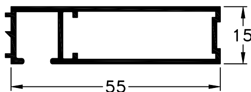
648 - Premarco Largo Std.: 6150 mm peso: 0,50 Kg/m
