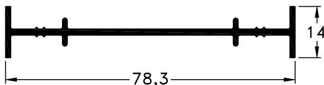
453 - Acople peso: 0,45 Kg/m
