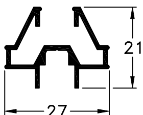
470 - Perimetral peso: 0,27 Kg/m
