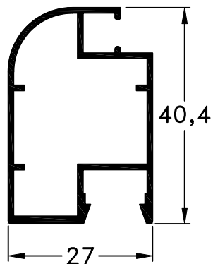
109 - Mosquitero peso: 0,44 Kg/m
