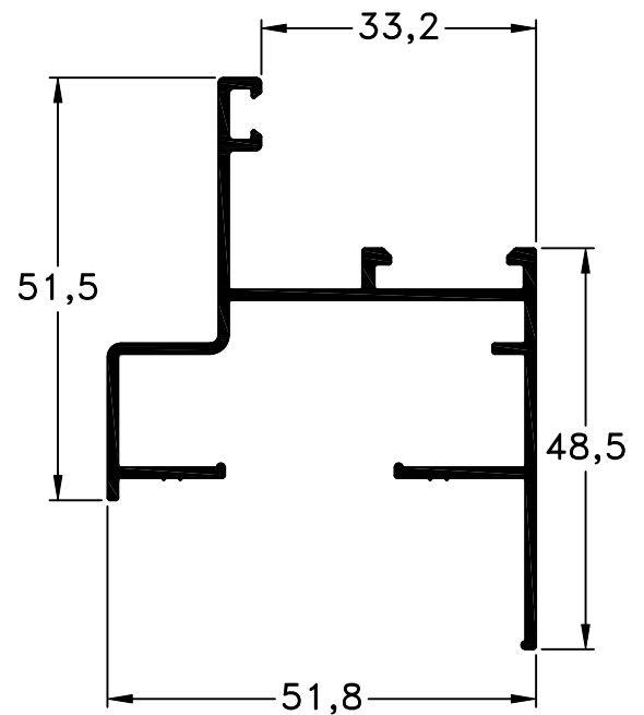
70 - Marco Paño Fijos y Ventana Doble Contacto Largo Std.: 6150 mm peso: 0,71 Kg/m
