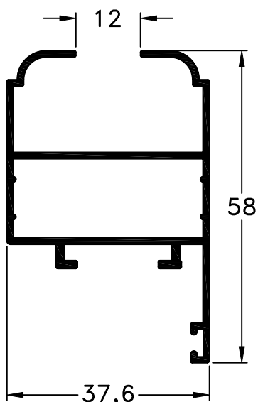
20 - Hoja peso: 0,68 Kg/m
