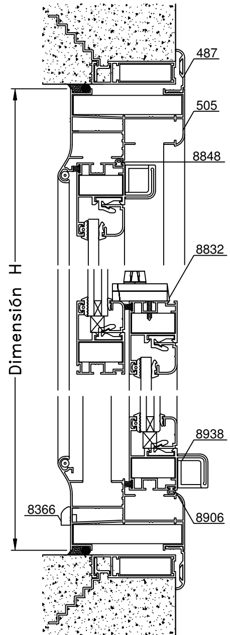
B-B Corte Vertical
