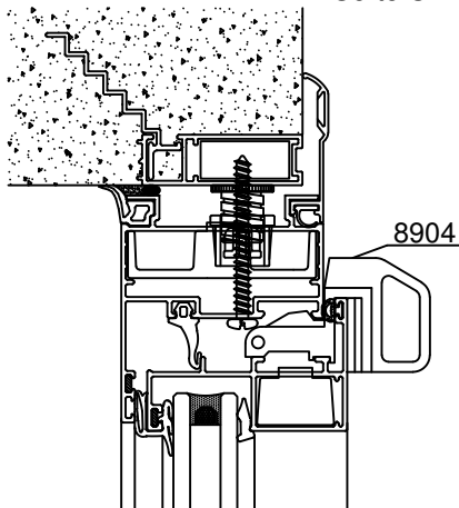
Corte C
